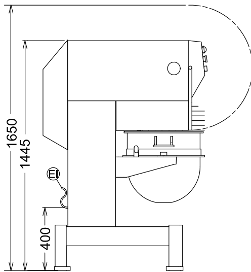
Zij aanzicht
